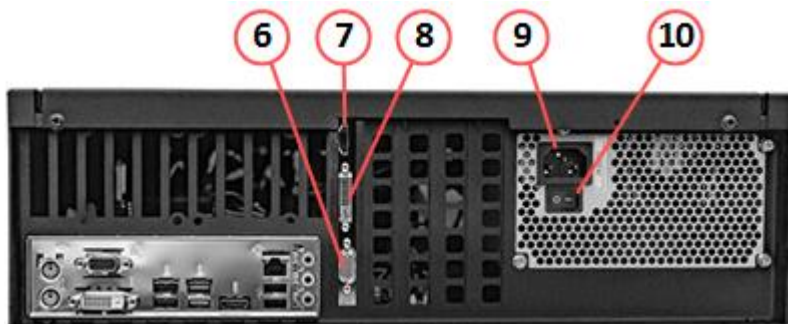
Рисунок 2. Задняя панель
