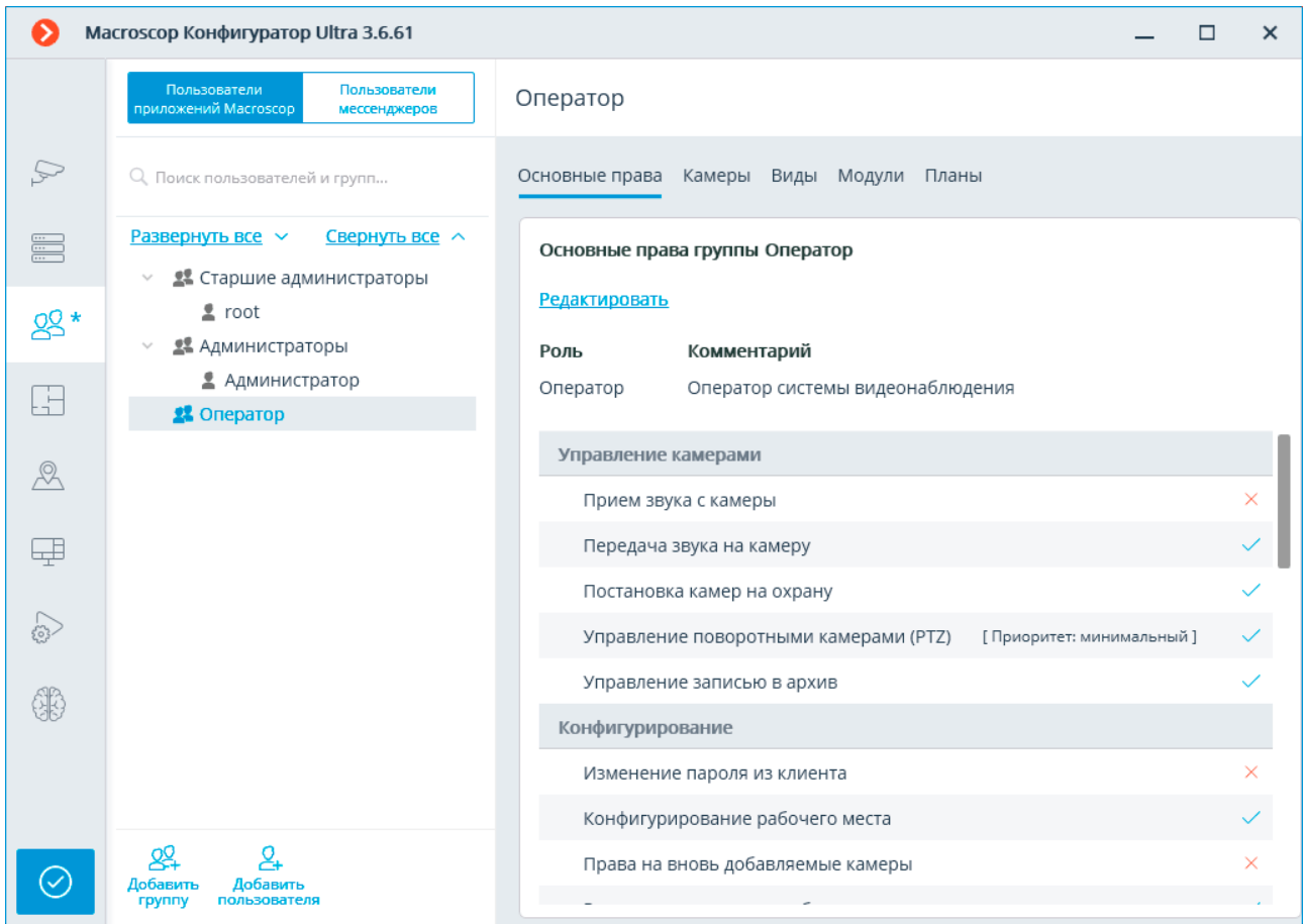
Групповое изменение основных прав
