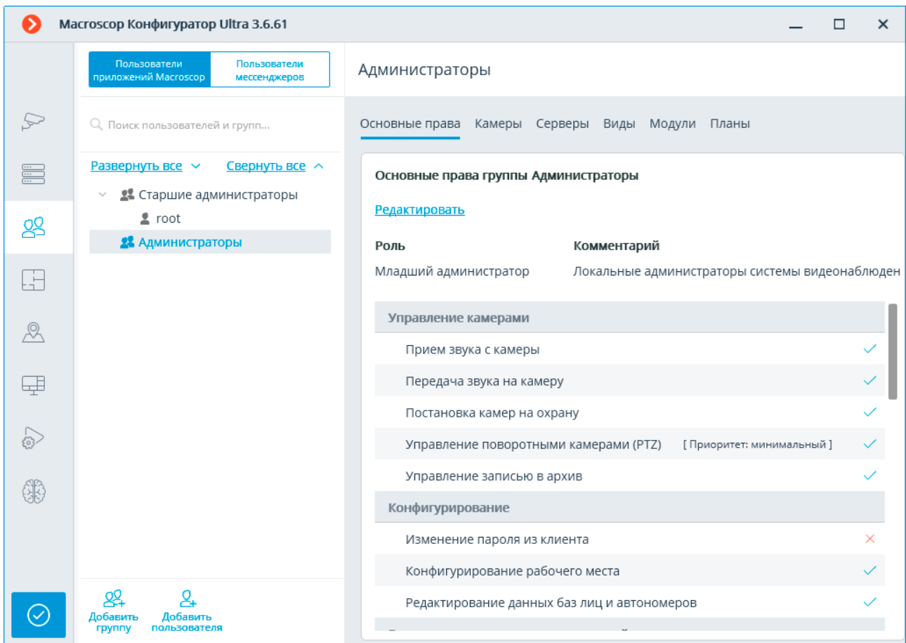
Предоставление прав на конфигурирование серверов
