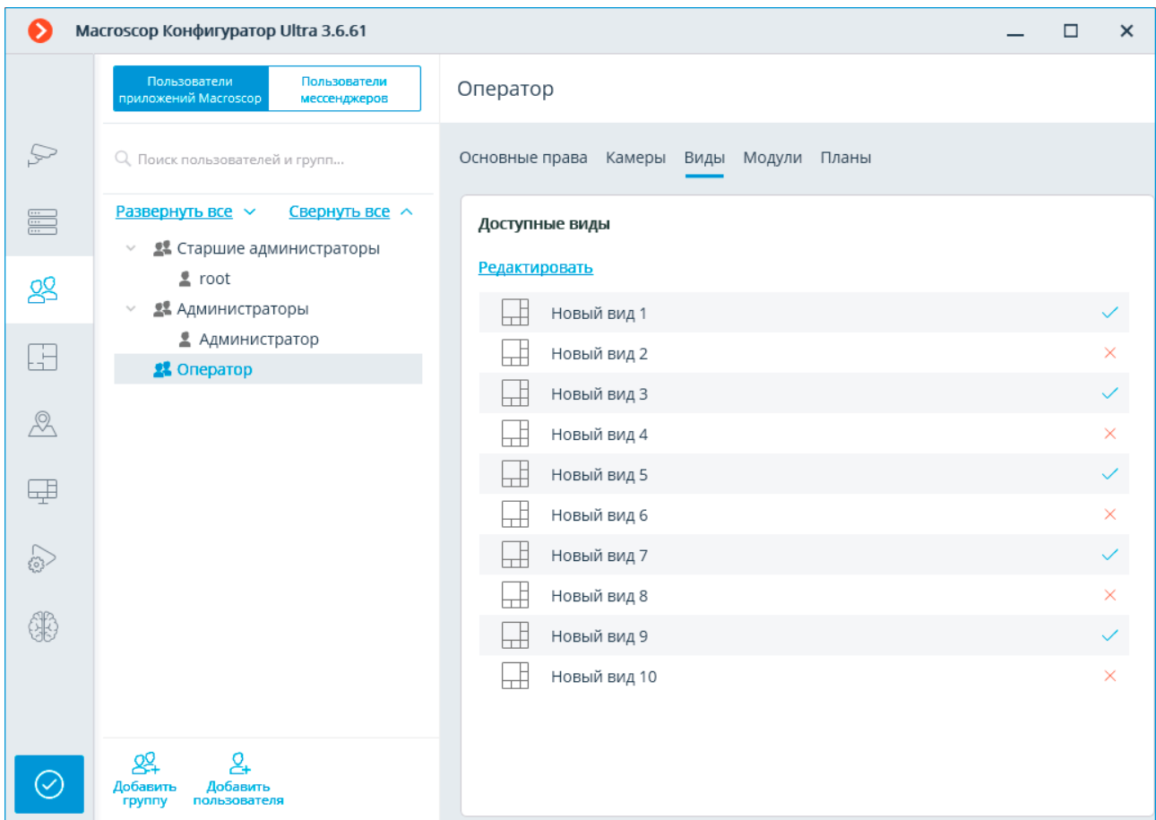
Изменение прав на использование модулей аналитики
