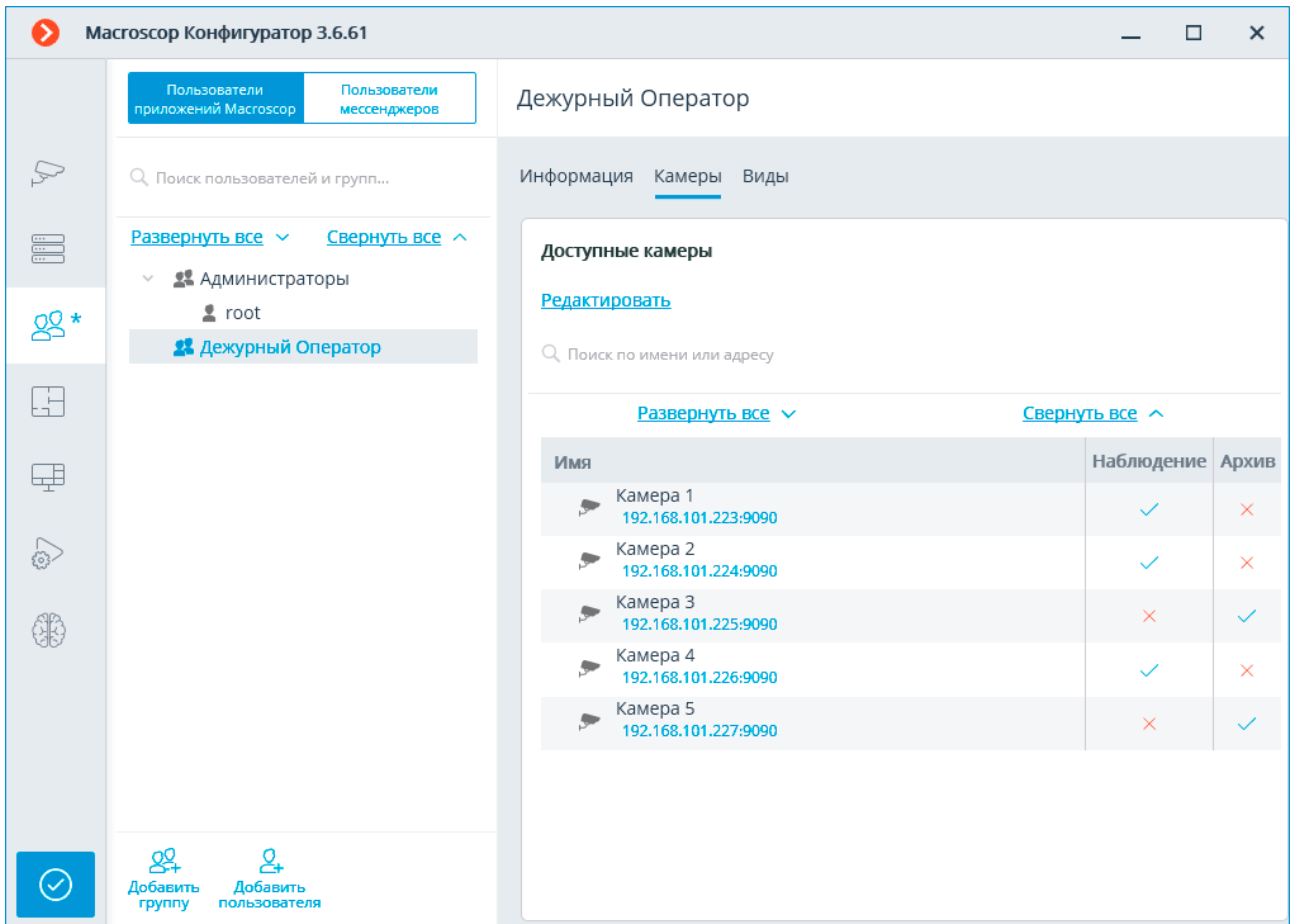
Групповое изменение прав на просмотр камер
