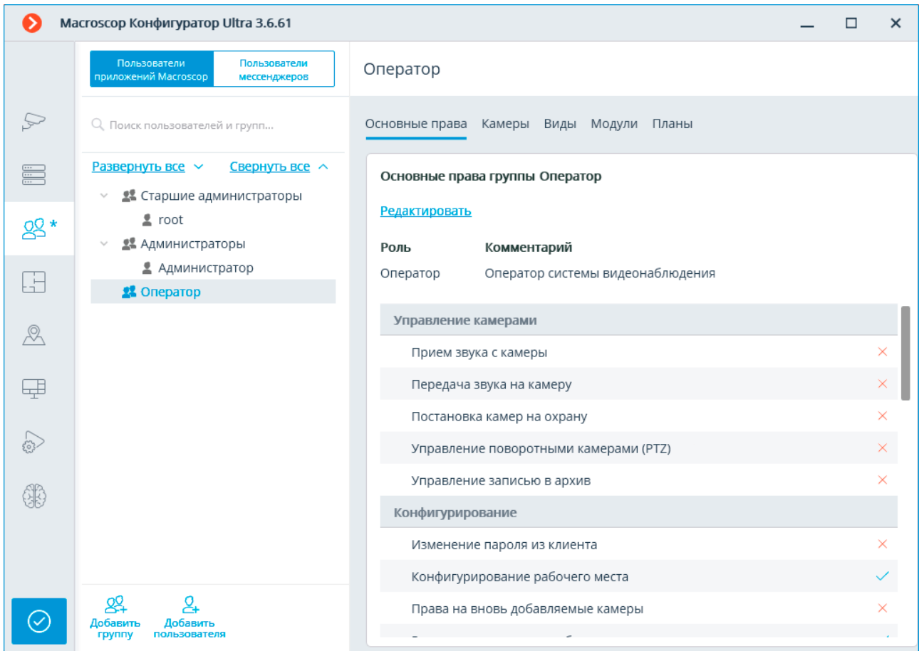
Изменение индивидуального права на просмотр камеры
