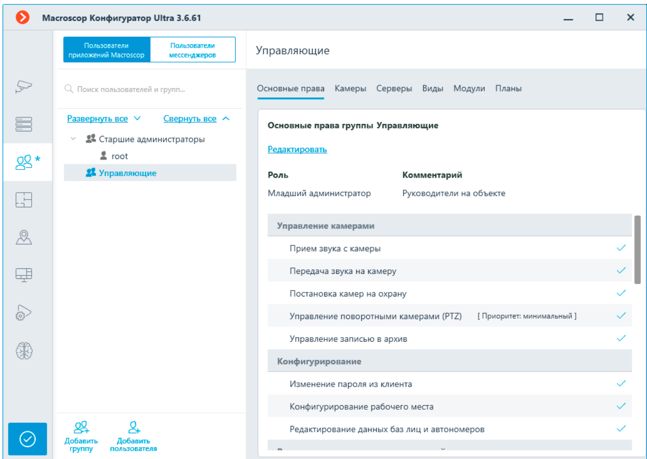
Изменение индивидуального основного права
